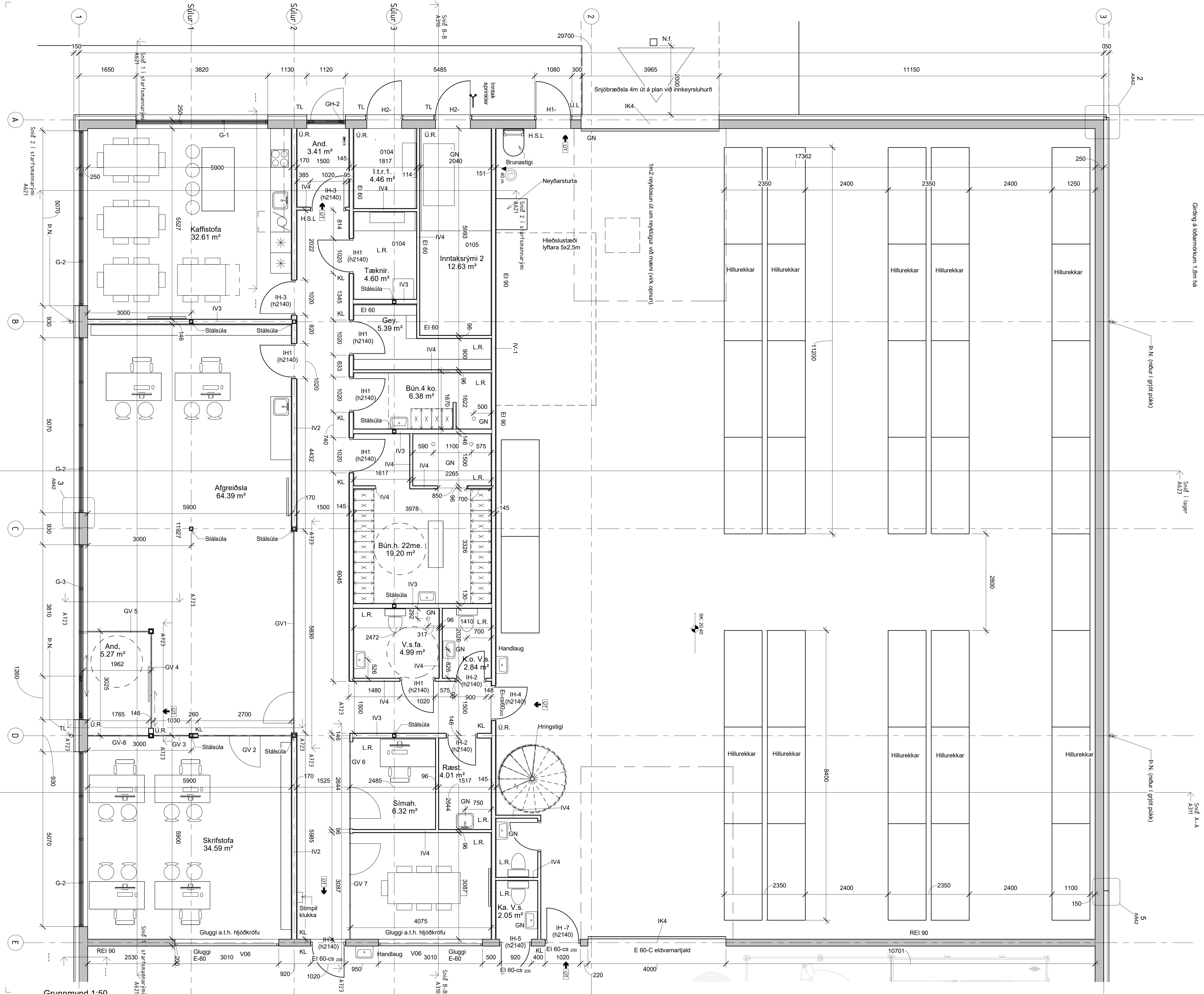
Grunnmynd 1:50
